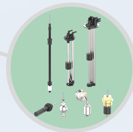
Füllstandsmessung
